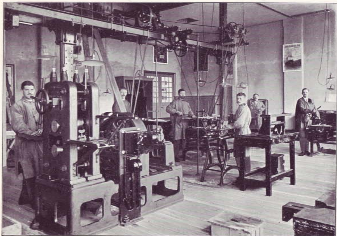
Lokaal voor de vervaardiging van Koperen Lijnen en Koperen Siermateriaal
