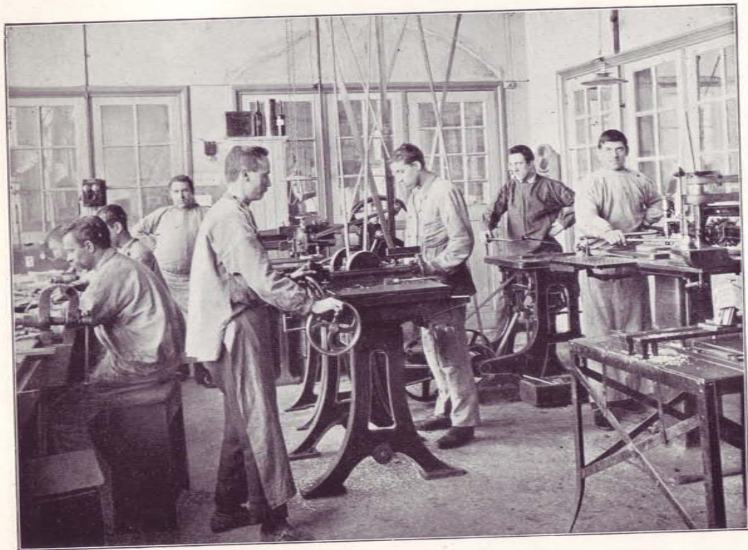
Lokaal voor mechanische afwerking van Galvano's en Stereotypen
